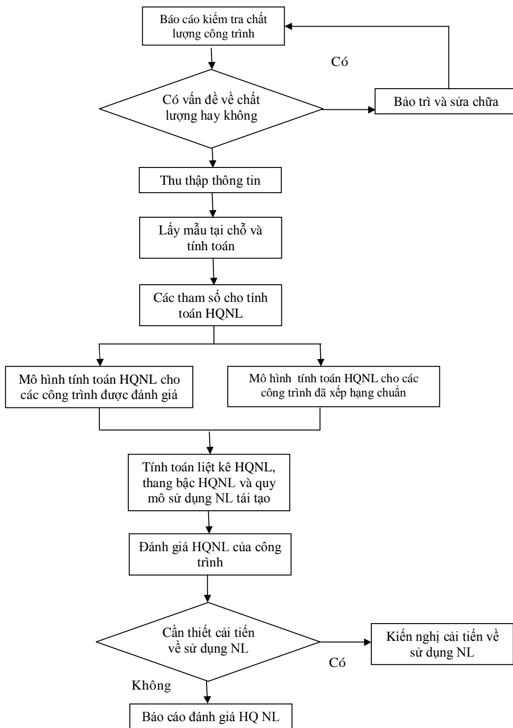
Hình 1. Quy trình đánh giá hiệu quả năng lượng (HQNL) cho các công trình dân dụng hiện hữu
