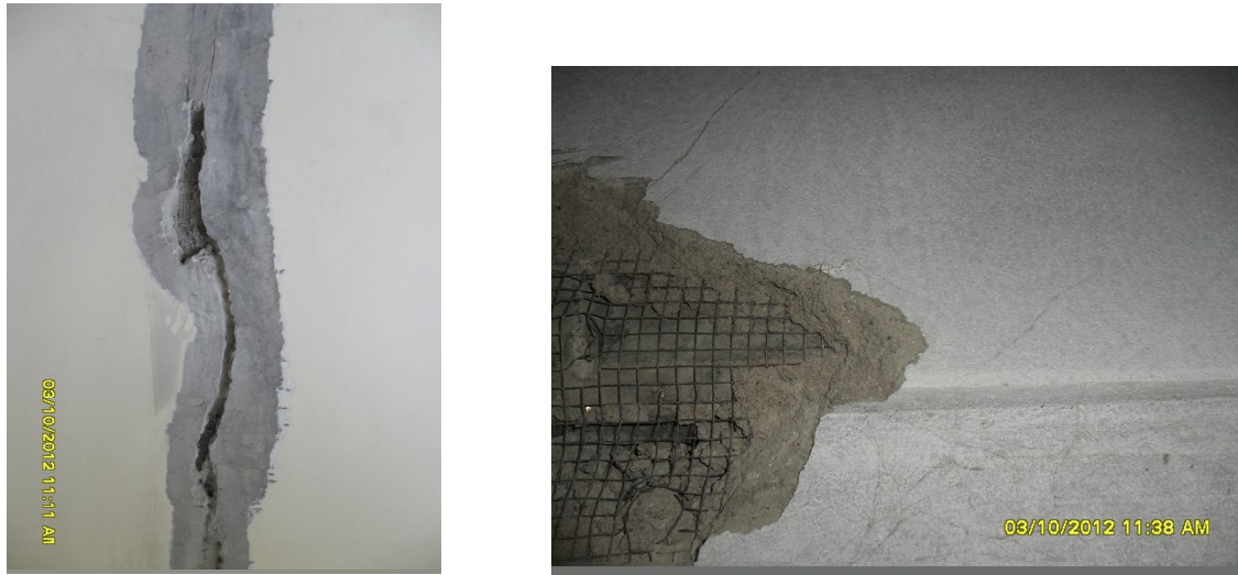
Hình 4. Nứt giữa vị trí tường xây với kết cấu chịu lực
