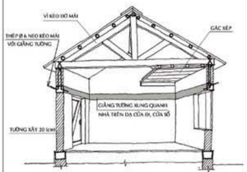
GIẢNG TƯỜNG Ở CAO ĐỘ CỬA ĐI, CỬA SỐ
