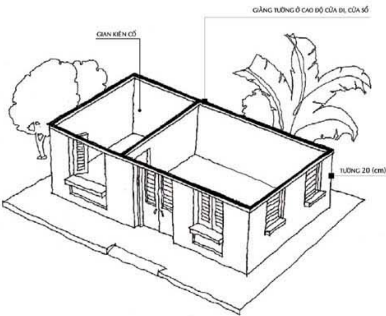
GIẢNG TƯỜNG XUNG QUANH NHÀ TRÊN ĐÁ CỬA ĐI, CỬA SỐ
