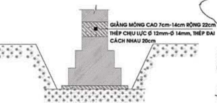
TRƯỜNG HỢP ĐẤT TỐT: ĐÁM KỶ NỀN TRƯỚC KHI XÂY MÓNG
