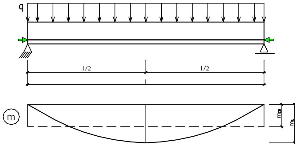
Hình 1: Sơ đồ dầm chịu tải trọng phân bố đều
