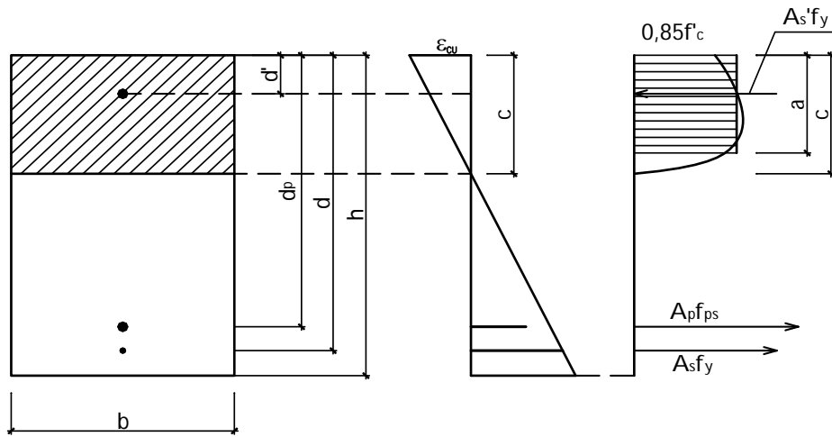
a) Sơ đồ mặt cắt dầm b) Sơ đồ biến dạng c) Sơ đồ ứng suất
