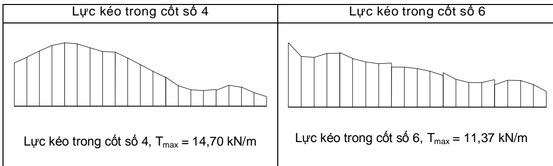
Hình 10. Lực kéo trong các cốt điển hình tại thời điểm cuối cùng
