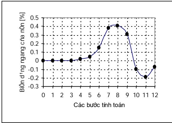
Hình 3. Biến dạng ngang của nền trong quá trình khai thác
