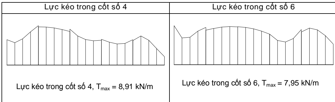
Hình 9. Lực kéo trong các cốt điển hình khi nền có biến dạng \varepsilon_{BC} = 0,4\%
