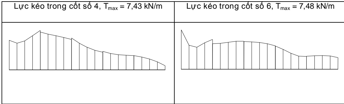
Hình 8. Lực kéo trong các cốt điển hình khi nền có biến dạng nhỏ \varepsilon_{BC} = 0,2\%
