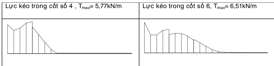
Hình 7. Giá trị lực kéo trong các cột điển hình trước khi có biến dạng nền
